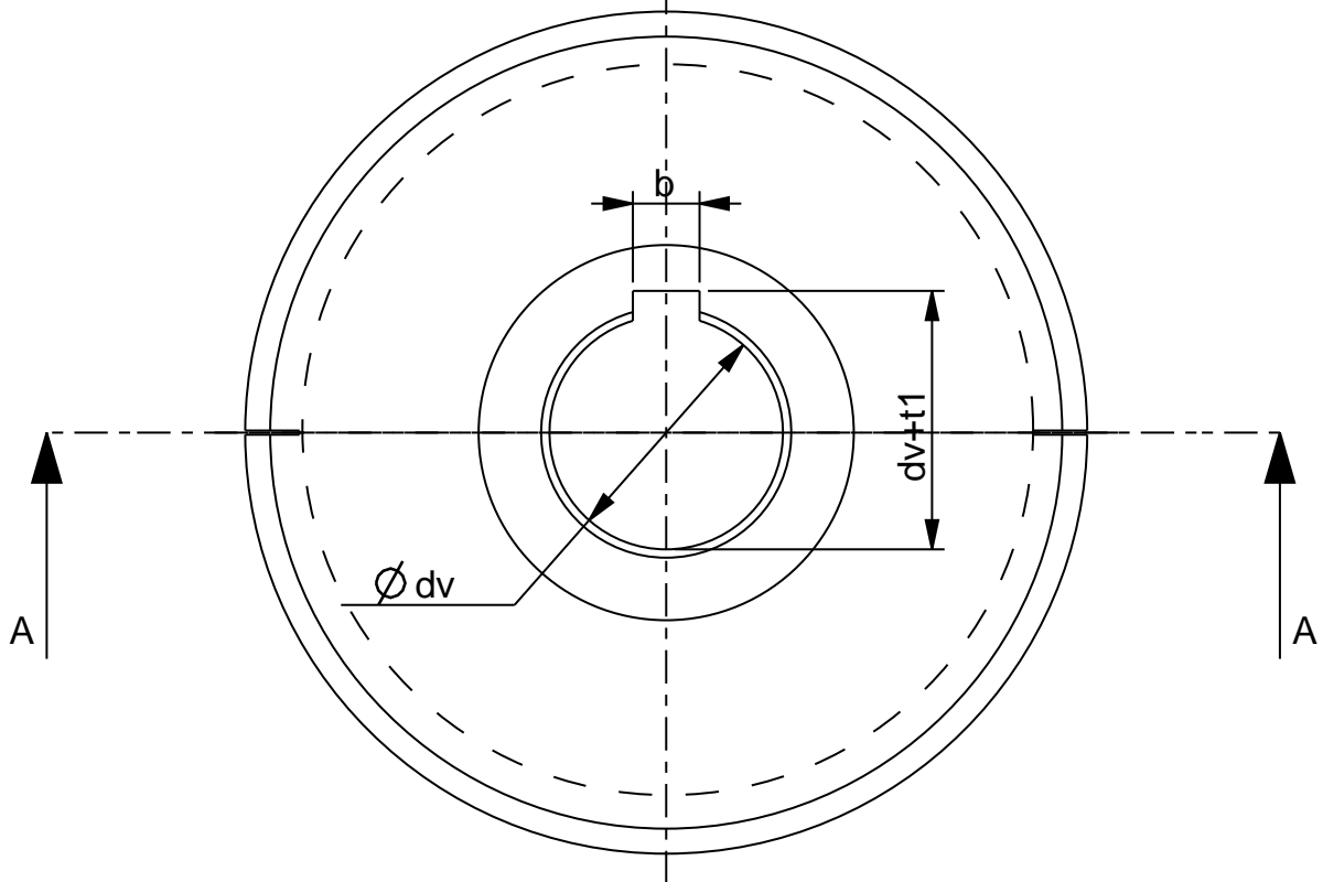
Presek A-A
